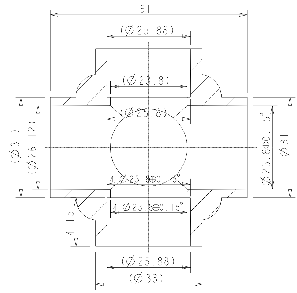
A-A断面図
